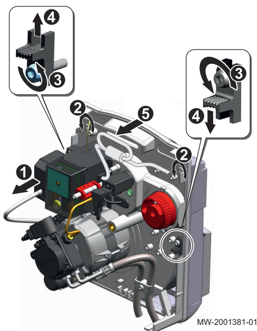
Afb.118 Verstuiver vervangen
