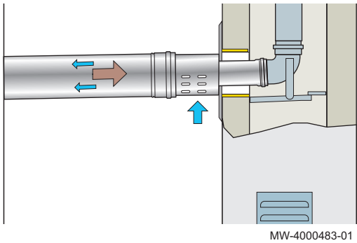
Afb.39 Type B 23P aansluiting – van toepassing binnenshuis in Frankrijk
